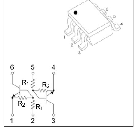
SOT-363
