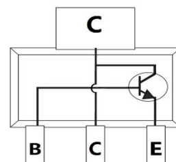
SOT-223
