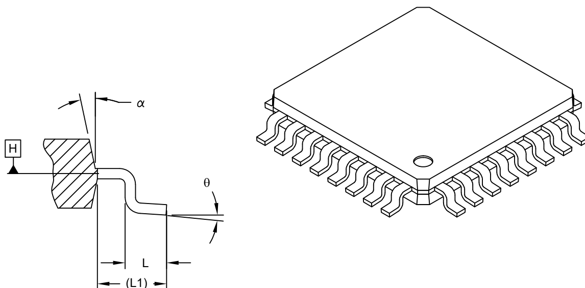
SECTION A-A
