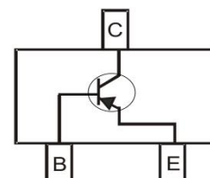
SOT-323
