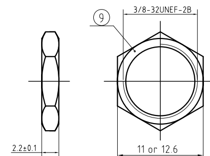
HEX NUT
