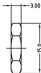
METAL NUT
