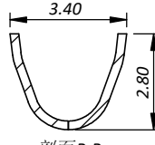
剖面 B-B 比例 5:1
