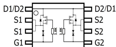
TSSOP-8
