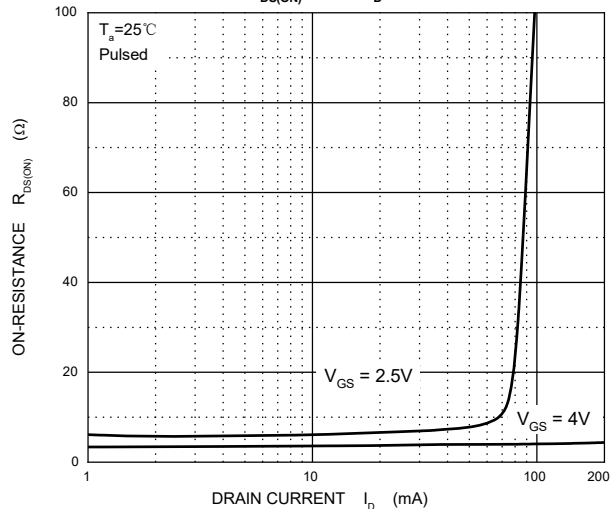
R_{DS(ON)} — I_D
