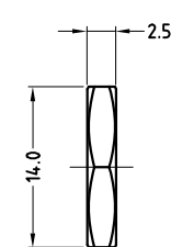
METAL NUT
