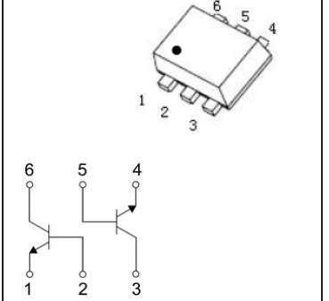
SOT-563
