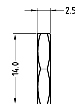
METAL NUT
