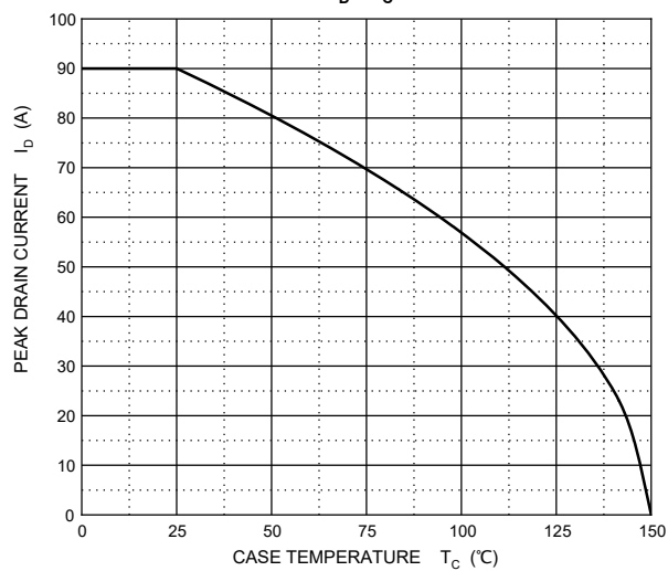
I_D - T_c
