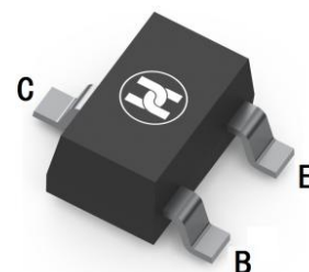
SOT-323
