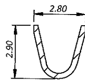
剖面 A-A 比例 5:1
