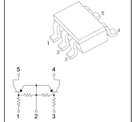
SOT-353
