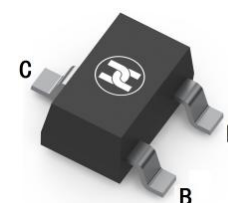
SOT-323
