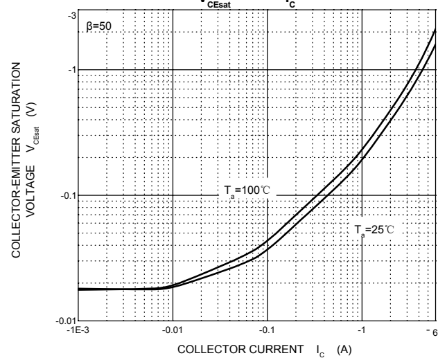
V_{CEsat} — I_c
