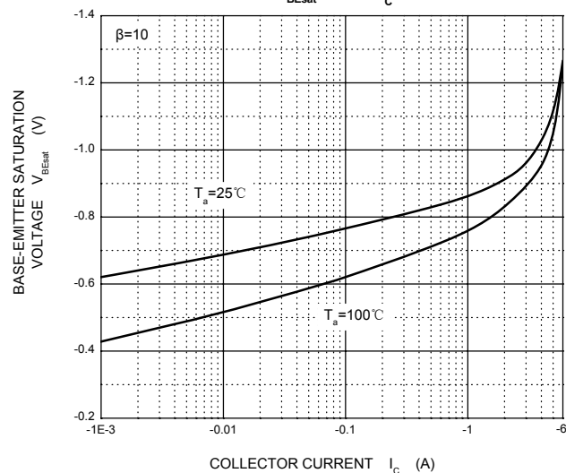
V_{BEsat} — I_c
