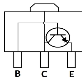
SOT-89
