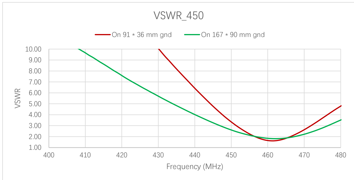
VSWR
