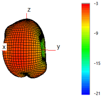
412 MHz
