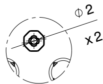
Det D (position pin)
