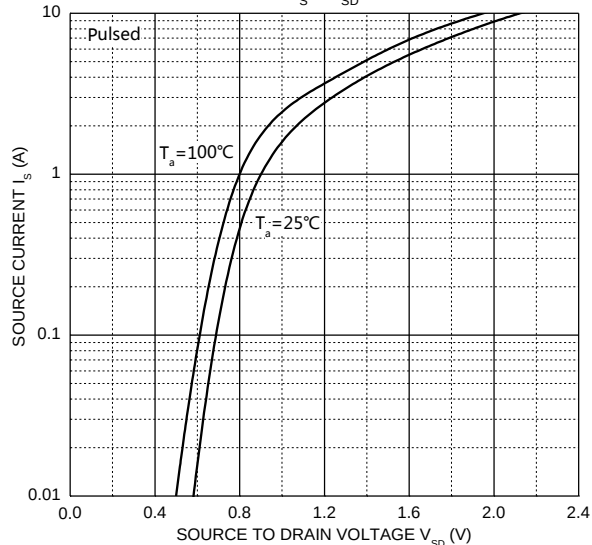
I_S - V_{SD}
