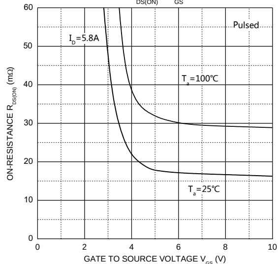
R_{DS(ON)} - V_{GS}
