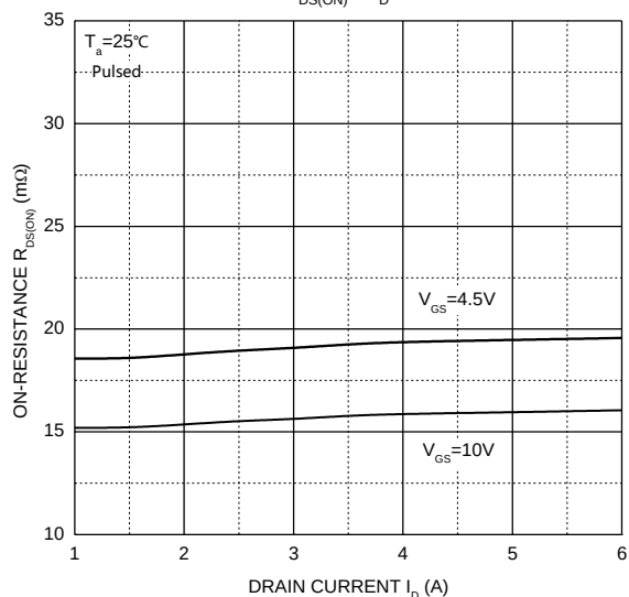
R_{DS(ON)} - I_D
